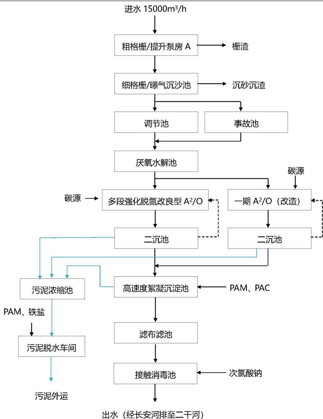
图 4-2 柘塘污水处理厂污水处理工艺流程图
