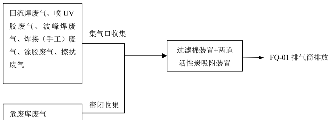
图 4-1 项目废气收集、治理路线图
