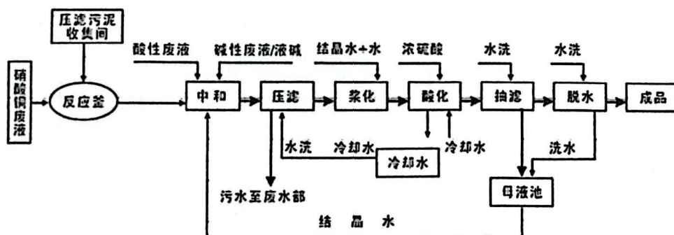
生产工艺流程图
