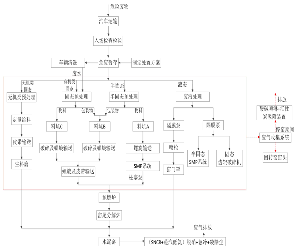
图 2-12 江苏中天共康环保科技有限公司原有项目生产工艺流程图
