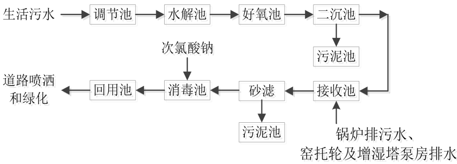
图 4-5 污水处理设备处理工艺流程图
