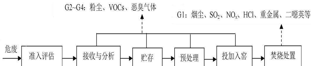
图 2-11 危险废物协同处置总体流程图
