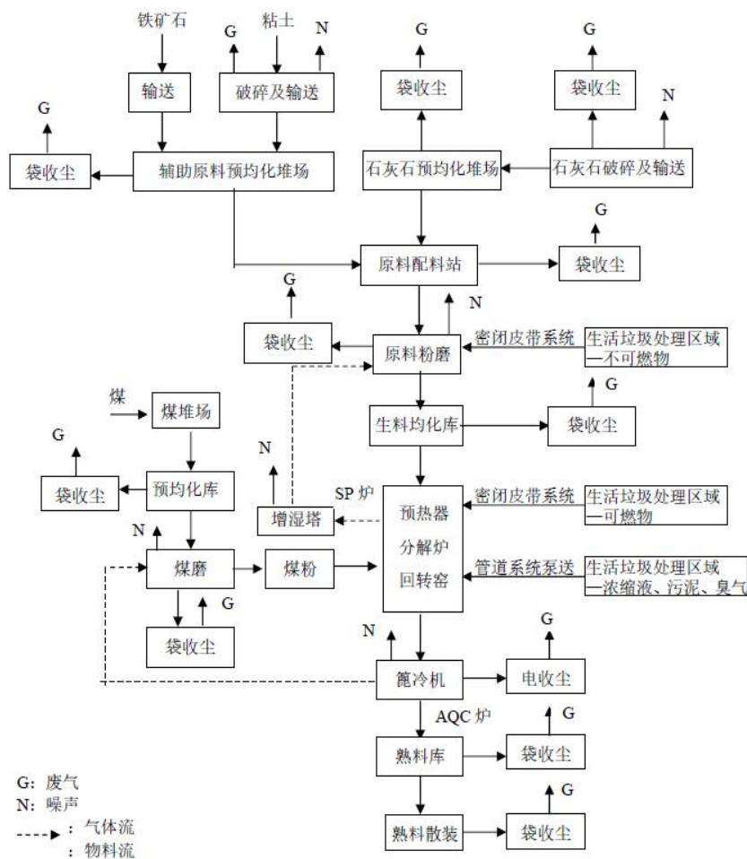
图 2-10 江苏省溧水天山水泥有限公司原有项目（与本项目有关）生产工艺流程图
