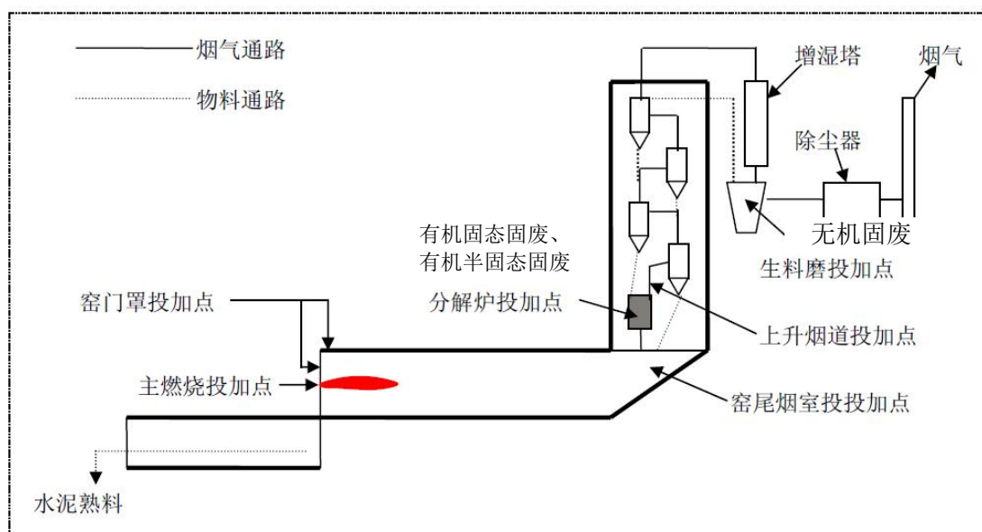
图 2-7 回转窑燃烧过程及可用于投料的位置
