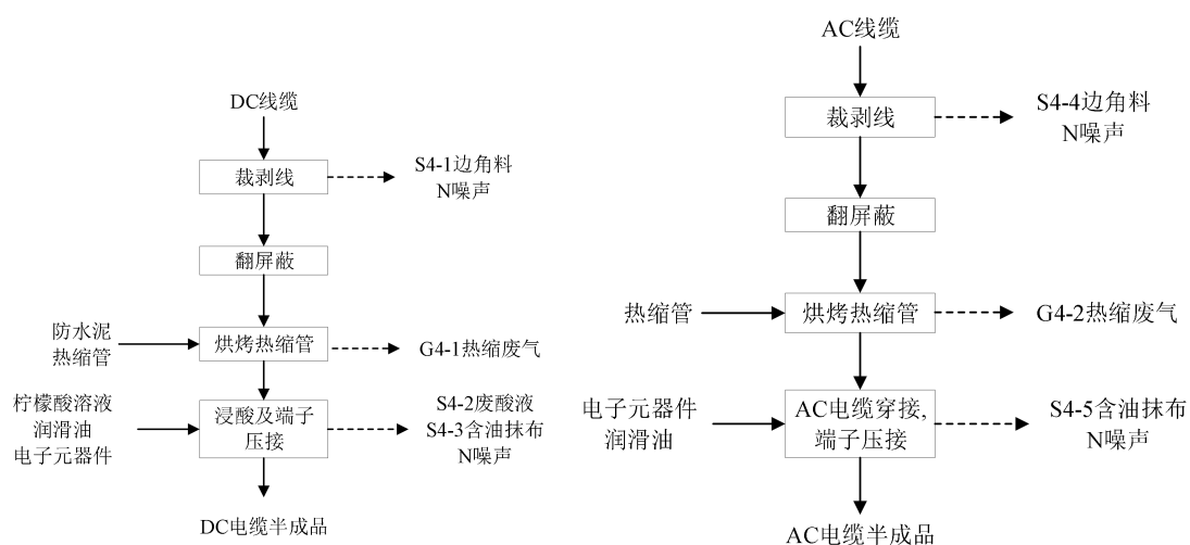
①DC 线缆半成品生产工艺流程图
