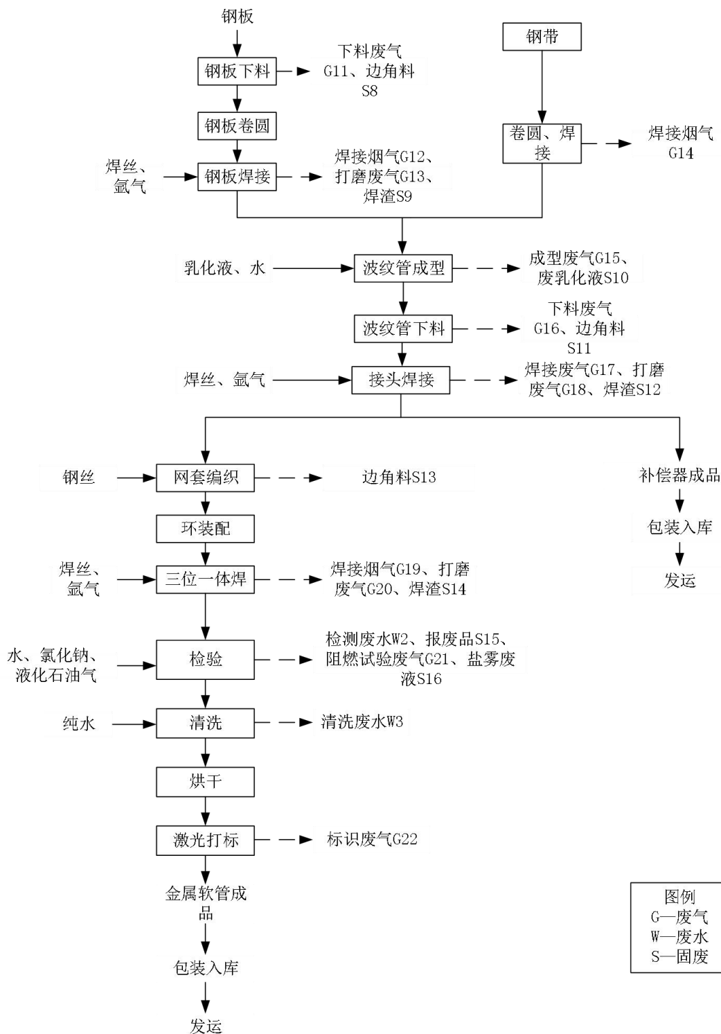
图 2-4 金属软管、补偿器生产工艺流程图
