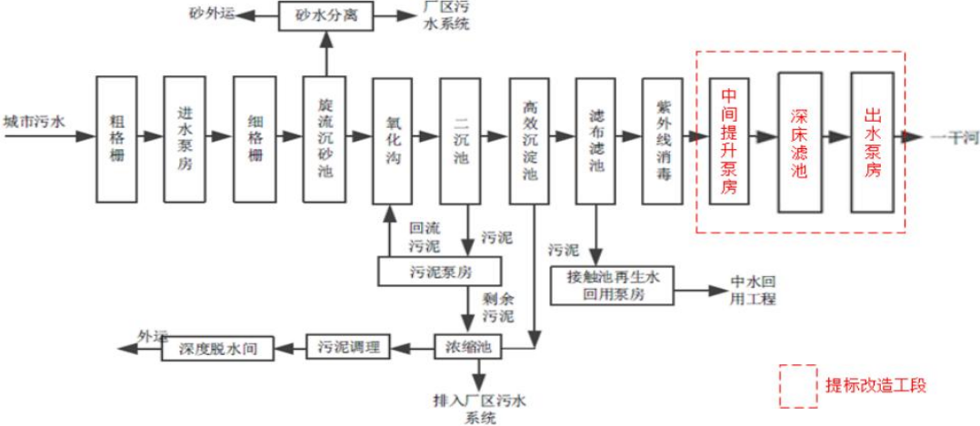
图 4-2 南京溧水秦源污水处理有限公司处理工艺流程图（一、二期）
