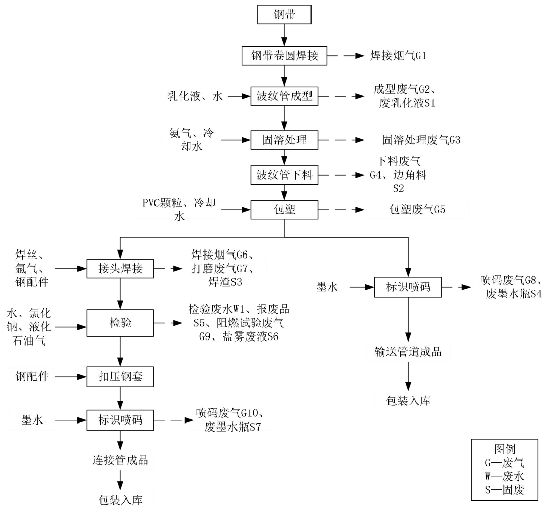
图 2-3 燃气连接管、燃气输送管生产工艺流程图
