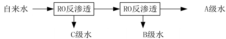
图 2-5 纯净水制备工艺
