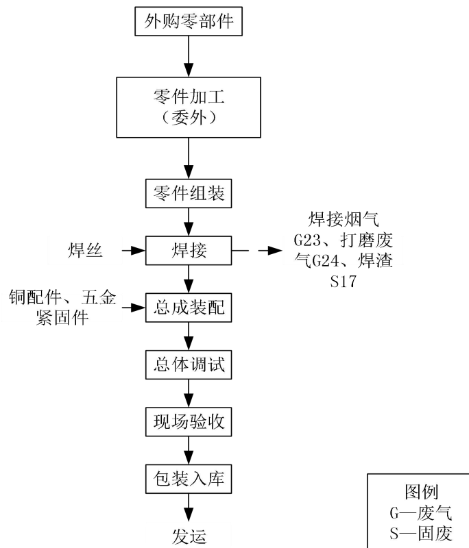
图 2-6 核电设备生产工艺流程图
