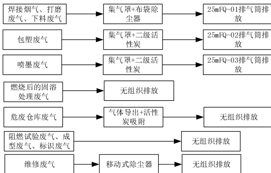
图 4-1 运营期废气治理措施图
