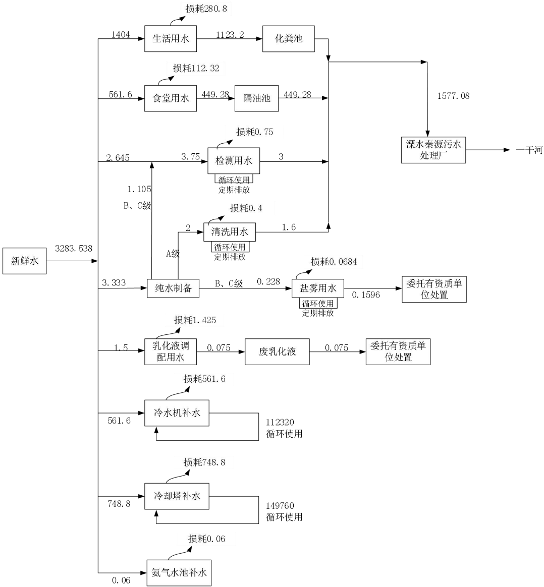
图 2-1 水平衡图 (t/a)
