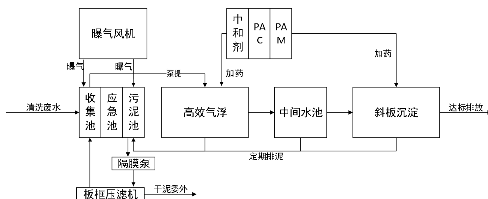
图 4-2 项目污水处理站处理工艺流程图
