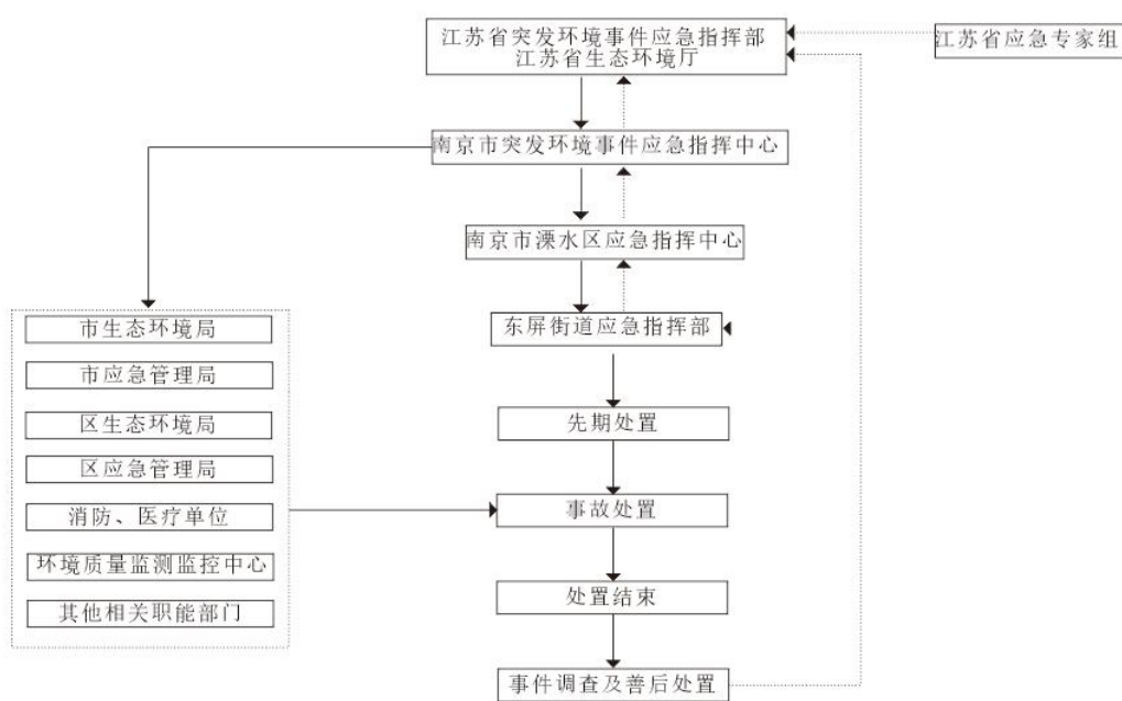
图6.2.3-3 重大及特别重大环境事件（II、I级）应急响应程序
