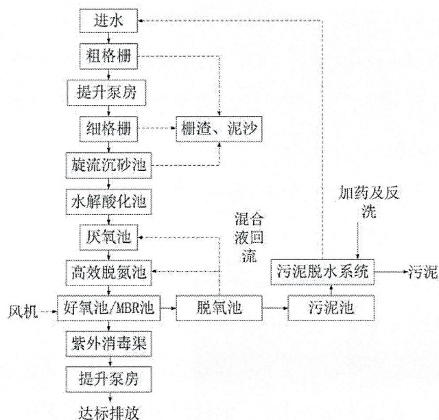
图 4-2 东屏污水处理厂处理工艺流程图
