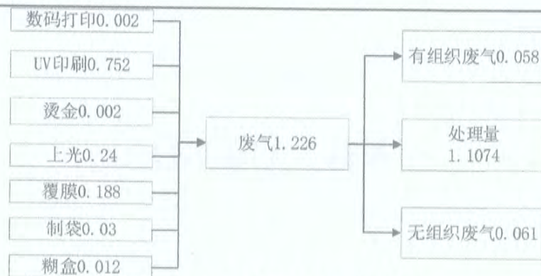
图 2-3 项目 VOCs 平衡图
