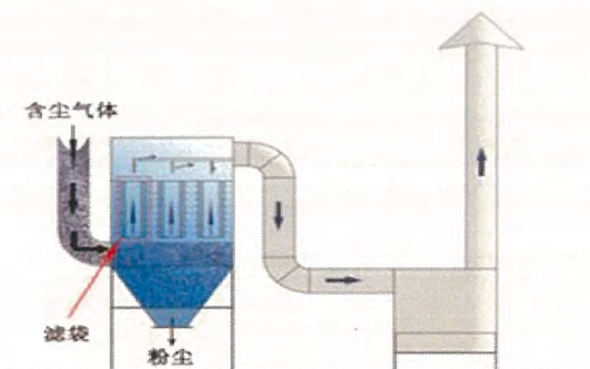
图 4-2 布袋除尘器效果图
