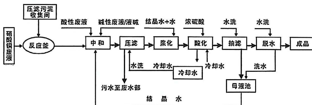
生产工艺流程图
