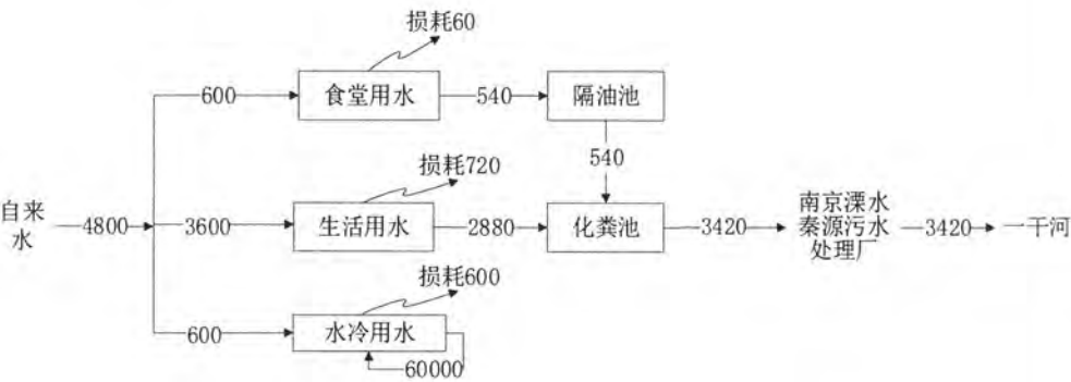
图 2-2 项目水平衡图 (t/a)
