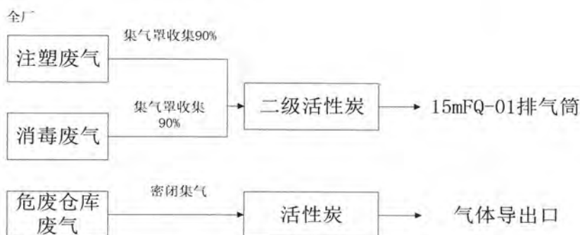
图 4-1 废气处理工艺流程图
