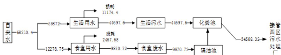
图 2-7 现有 3 号地块水平衡图 单位 ( \text{m}^3/\text{a} )
