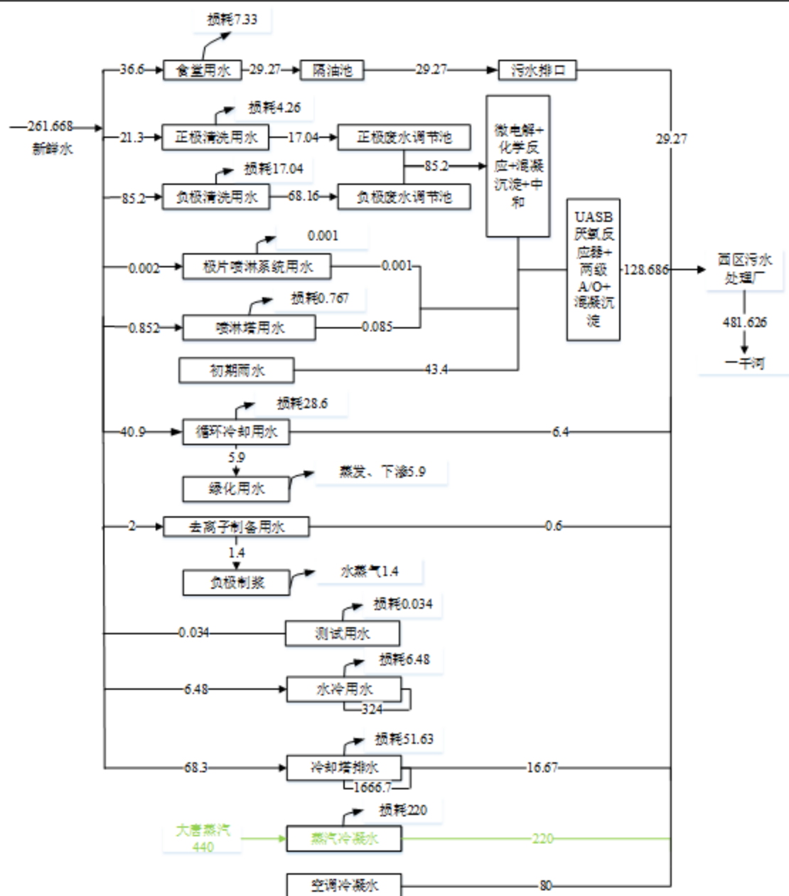
图 2-6 现有 1、2 号地块水（汽）平衡图 单位 ( \text{m}^3/\text{d} )
